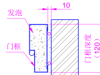
刚结构 连接节点图
