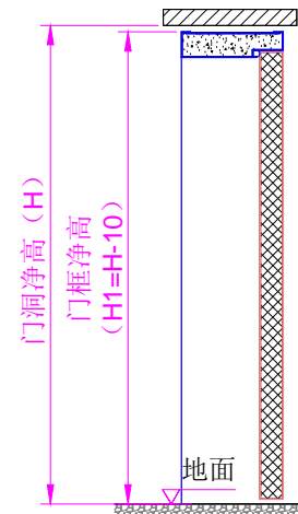
墙体连接节点图
