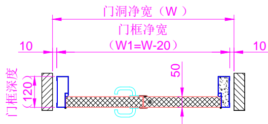
双开门剖面图
