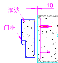
钢质门门框 连接节点图
