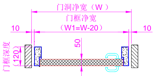
单开门剖面图
